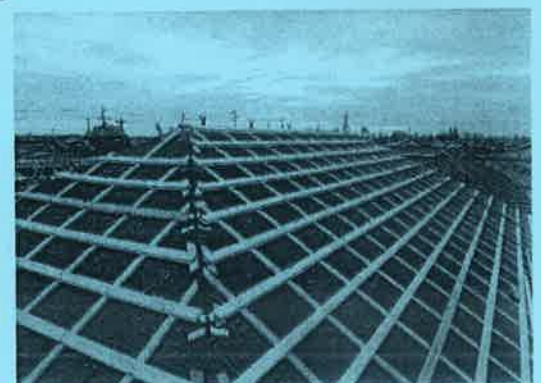
たて椽、よこ椽工法におり 水が抜ける仕組みをつくる
